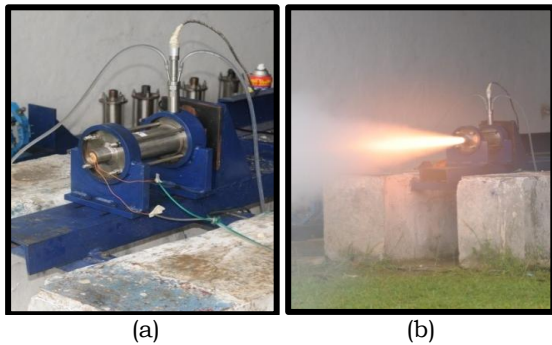
Gambar 3-10: (a) Motor roket terpasang pada load cell; (b) Proses pengujian statik
