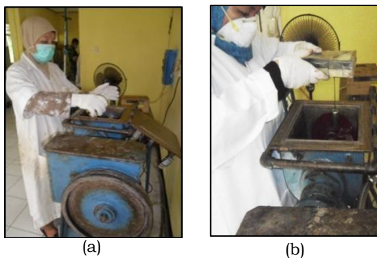
Gambar 3-4: (a) Pemasukan bahan; (b) Pengukuran viskositas adonan propelan
