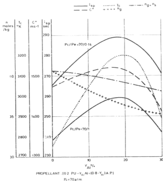
Gambar 4-1: Pengaruh kandungan fuel (Al) terhadap beberapa parameter
