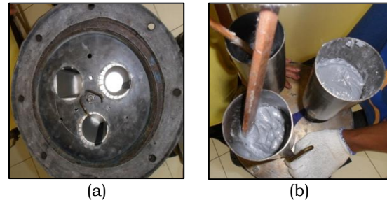
Gambar 3-5: (a) Tabung cetakan dalam vacuum casting chamber ; (b) Proses casting
