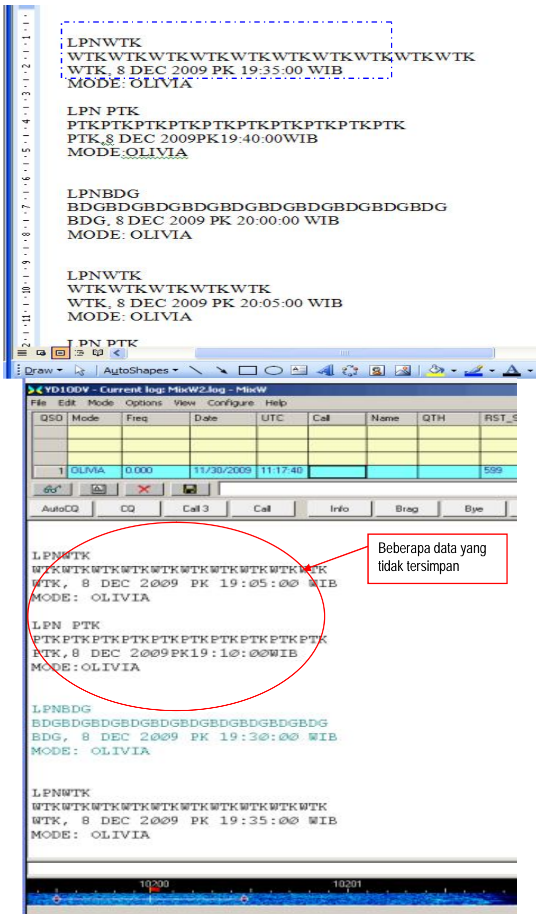
Gambar 4-1: Hasil pengamatan uji komunikasi radio pada tanggal 8 Desember 2009 dengan frekuensi kerja 10,200 MHz
