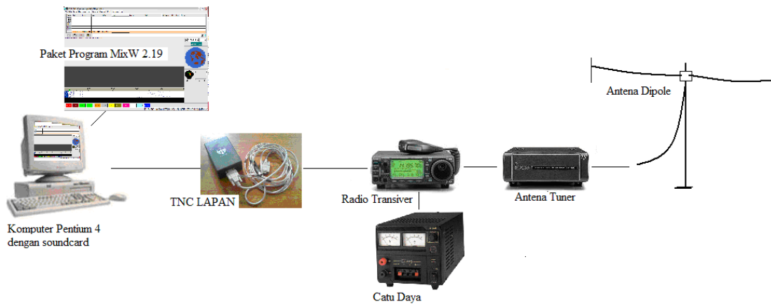
Gambar 2-1: Konfigurasi peralatan pengamatan
