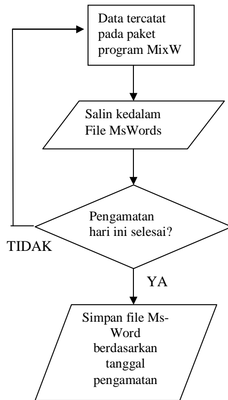
Gambar 2-3: Diagram alur proses penyimpanan data uji komunikasi radio
