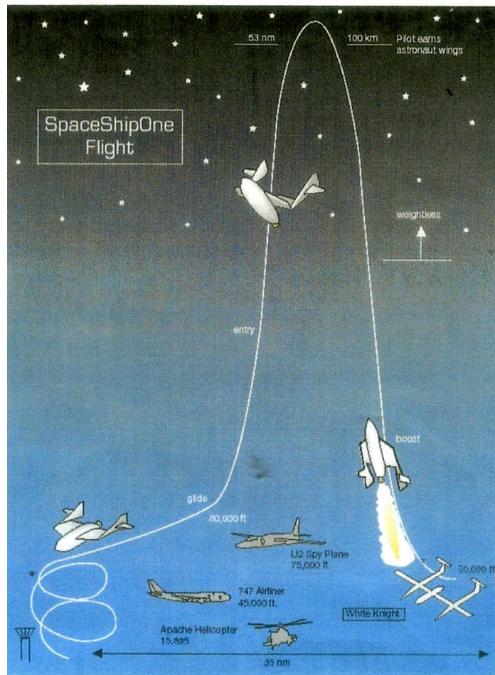
Gambar 5-1: Trayektori pesawat SS-1
