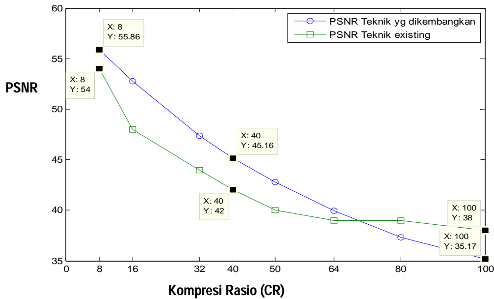
Gambar 4-3: Perbandingan teknik existing dengan Linier rata-rata (level dekomposisi wavelet = 3)
