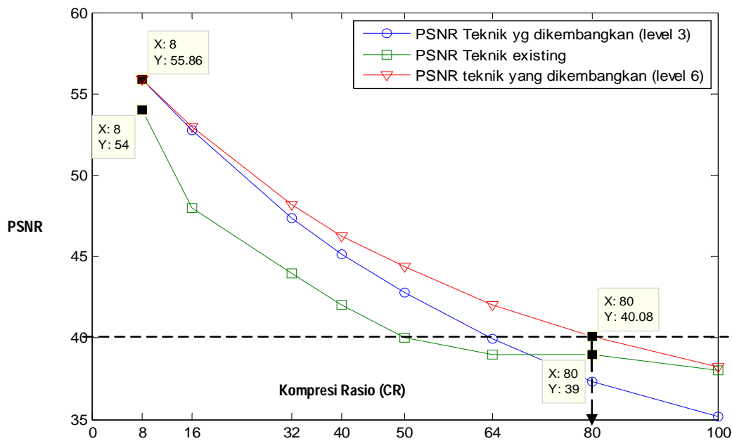
Gambar 4-4: Perbandingan Teknik Existing dengan Linier rata-rata terdekat (level dekomposisi wavelet = 6)
