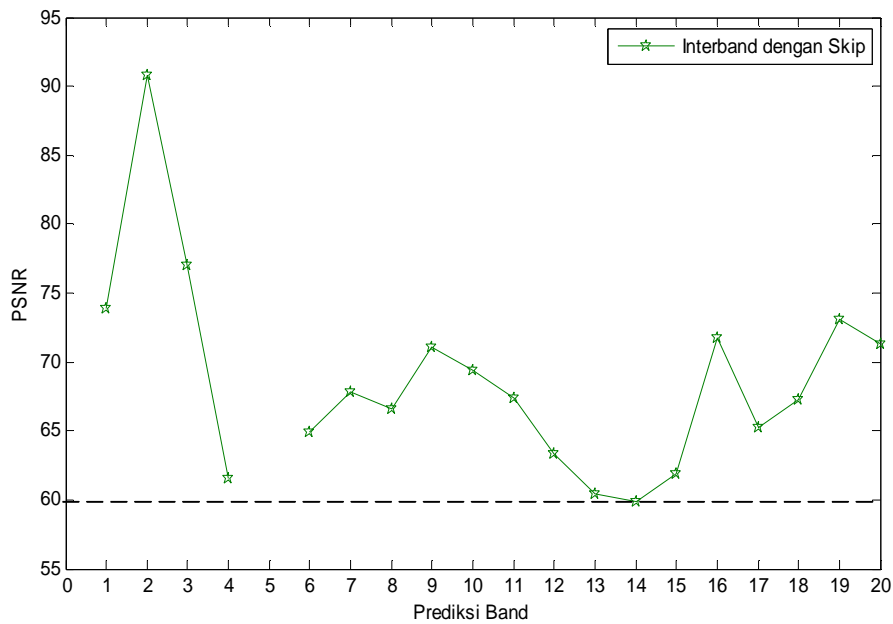
Gambar 4-2: Interkanal prediksi linier rata-rata terdekat dan skip citra kanal
