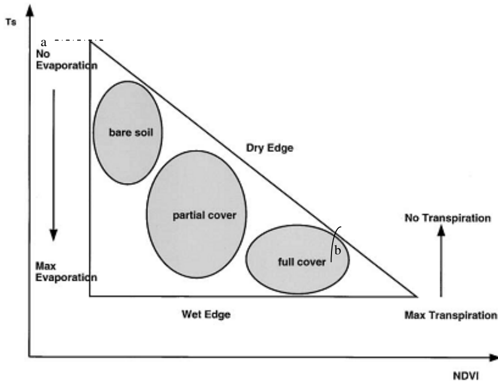
Gambar 2-1: Skema hubungan NDVI-Ts (Sandholt et al, 2002)
