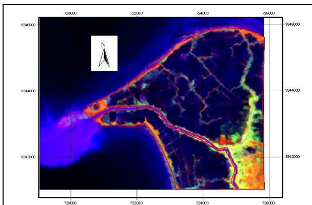
Gambar 4-1: Citra komposit RGB 453 Landsat-TM tahun 1990
