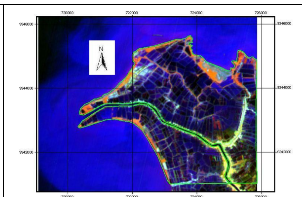
Gambar 4-2: Citra komposit RGB 143 SPOT-4 tahun 2007
