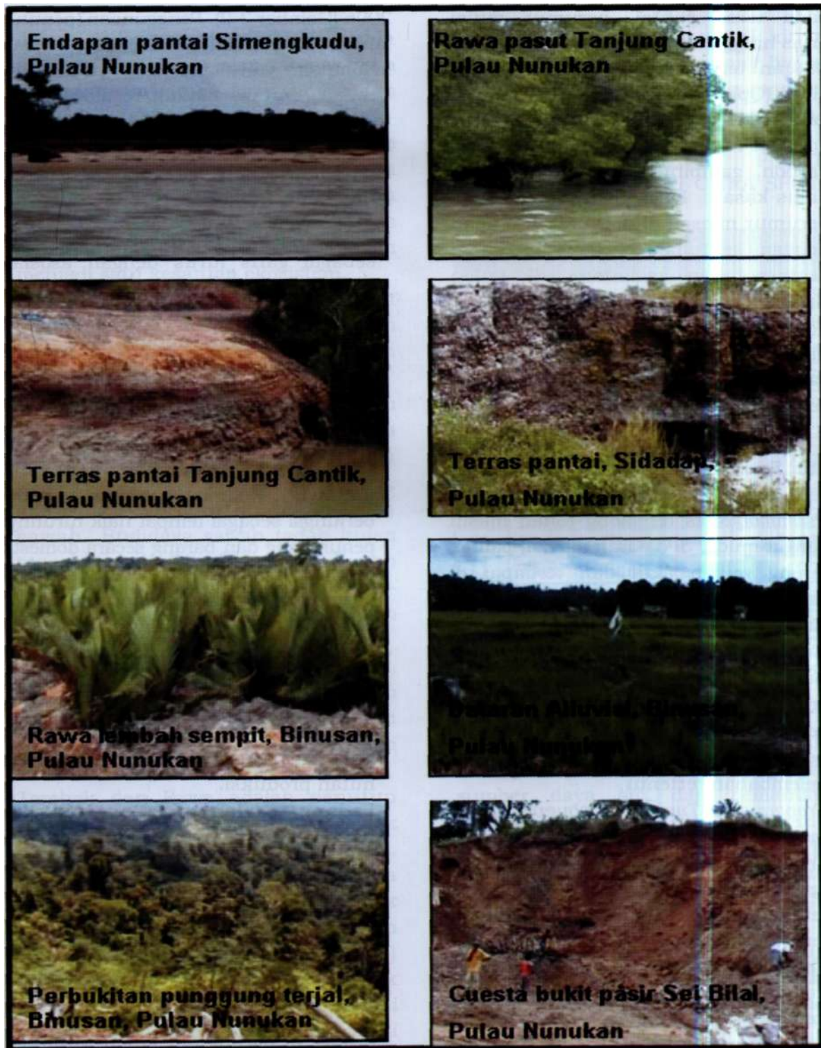
Gambar 3-1: Kenampakan bentuk lahan hasil survei lapangan Pulau Nunukan
