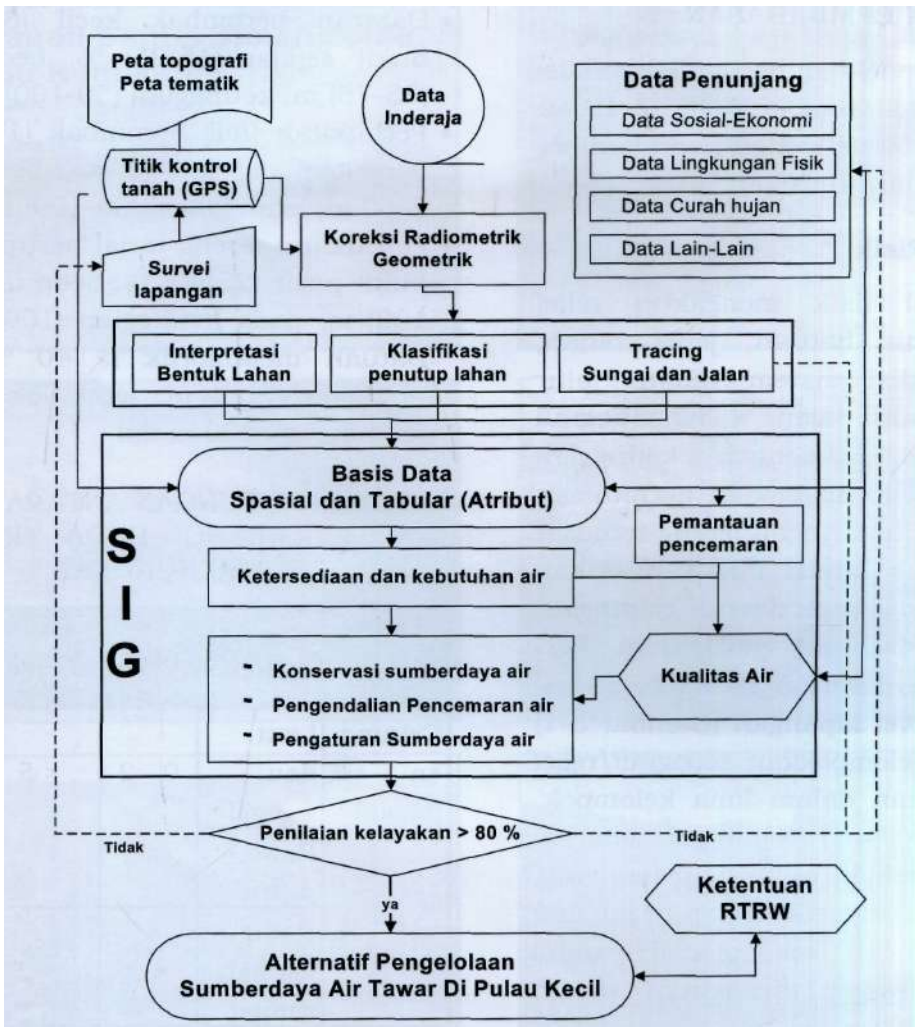
Gambar 2-1: Rancangan model analisis alternatif pengelolaan sumber daya air
