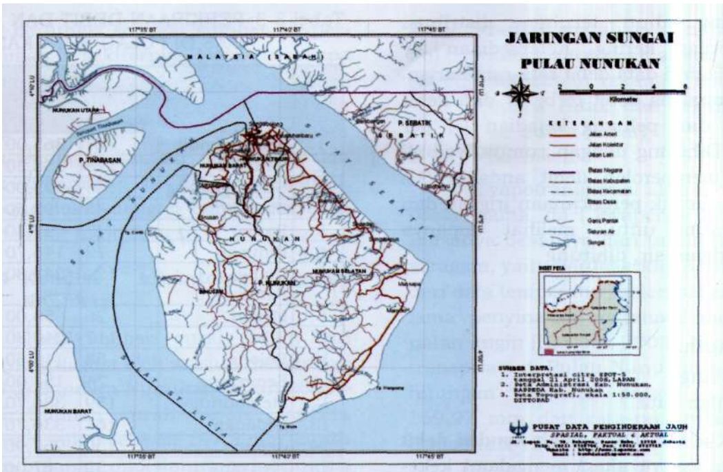
Gambar 3-3: Jaringan Sungai Pulau Nunukan Tahun 2006
