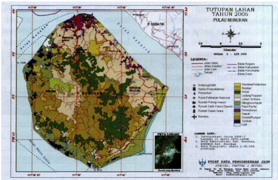
Gambar 3-2: Tutupan lahan Pulau Nunukan tahun 2006
