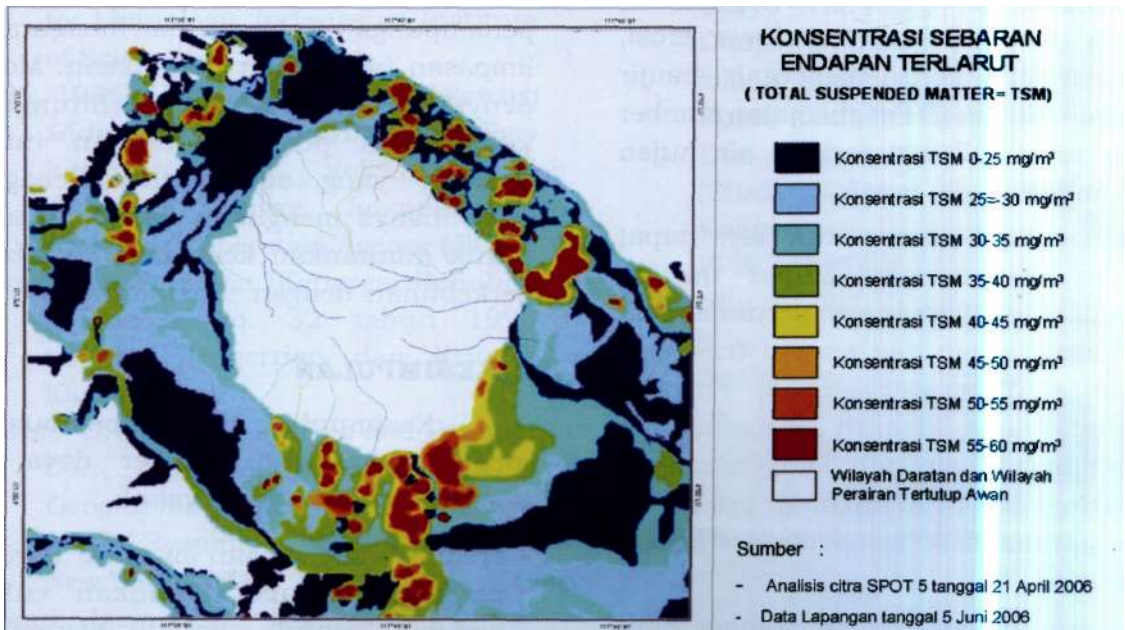
Gambar 3-4: Sebaran kandungan anorganik di perairan dan sungai di Pulau Nunukan dari citra SPOT 5 tanggal 21 April 2006
