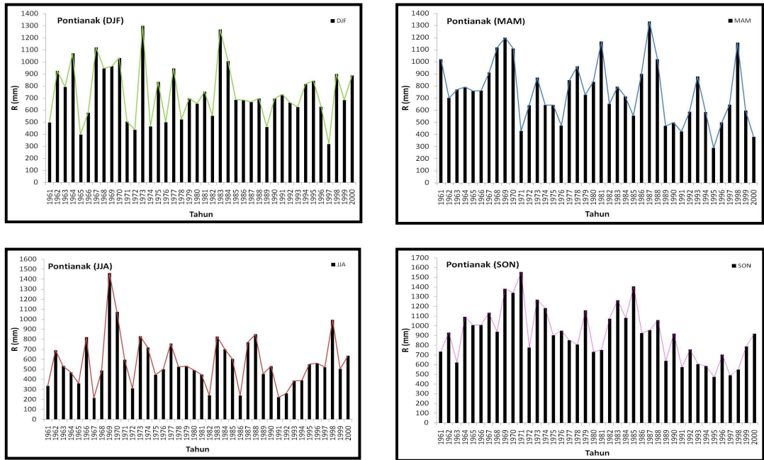
Gambar 3-1b: Jumlah curah hujan musiman DJF, MAM, JJA dan SON, Pontianak
