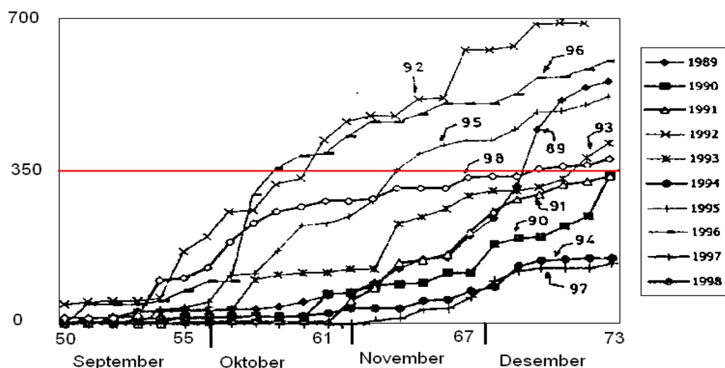
Gambar 3-2: Curah hujan kumulatif dari pentad ke 50 (3 September) sampai pentad ke 73 (31 Desember) di Jakarta
