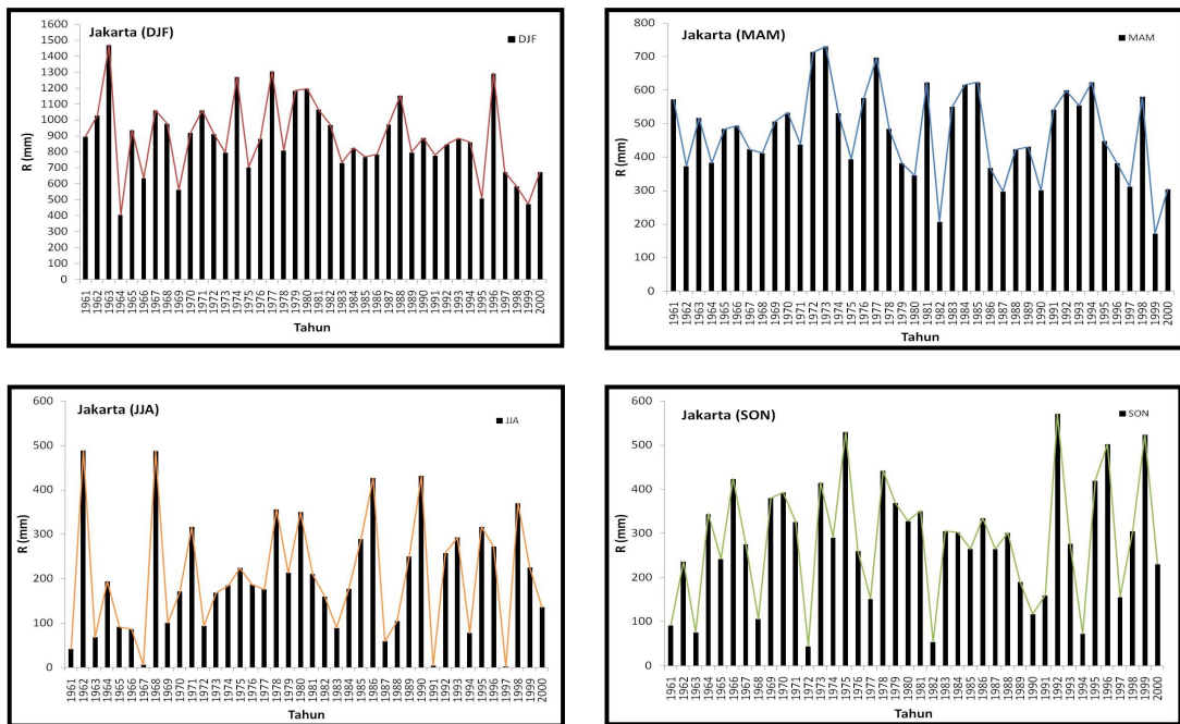
Gambar 3-1a: Jumlah curah hujan musiman DJF, MAM, JJA dan SON, Jakarta
