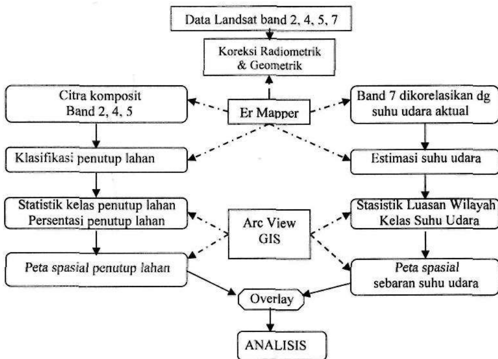
Gambar 2-1: Alur pemrosesan data citra Landsat sampai analisis
